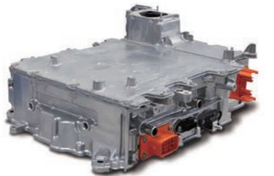
多合一集成电源单元
