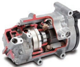
電動コンプレッサー ESBG27
