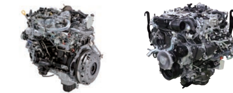
1GD-FTV型 排气量2.8L 搭载于兰德酷路泽250、 搭载于HIACE F33A-FTV型 排气量3.3L 搭载于兰德酷路泽300
