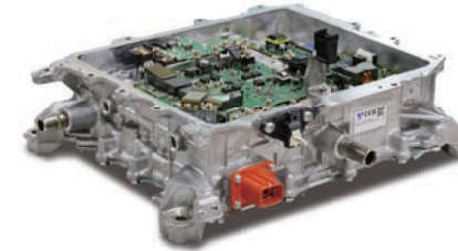
车载充电器、DC-DC 转换器 一体单元
