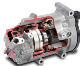
电动压缩机 ESBG27
