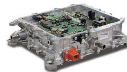
车载充电器、DC-DC 转换器 一体单元
